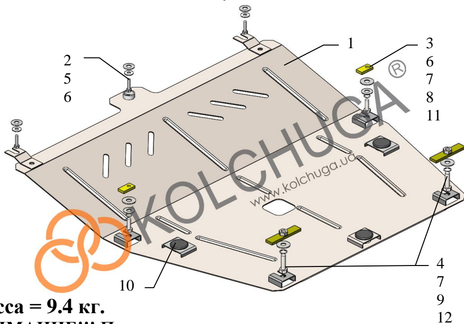
Схема установки.
