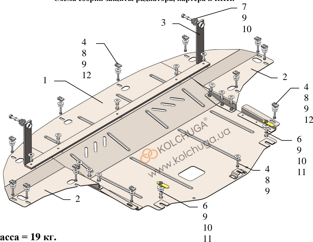
Схема сборки защиты радиатора, картера и КПП.
