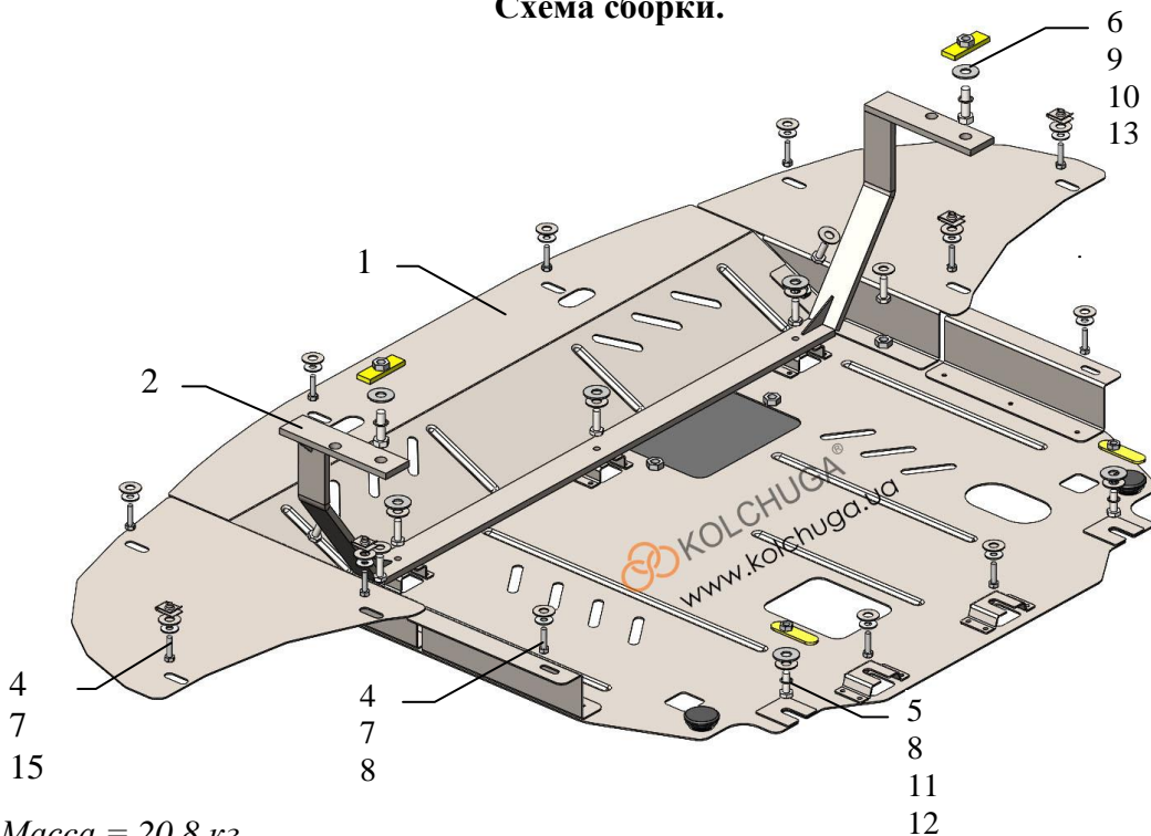
Схема сборки.
