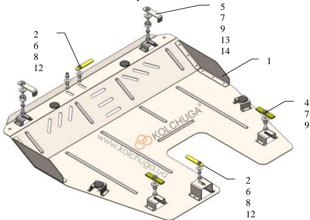
Схема установки.
