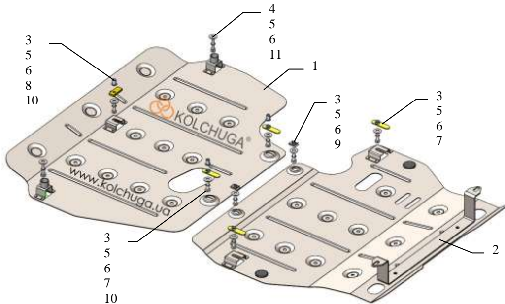
Схема сборки.
