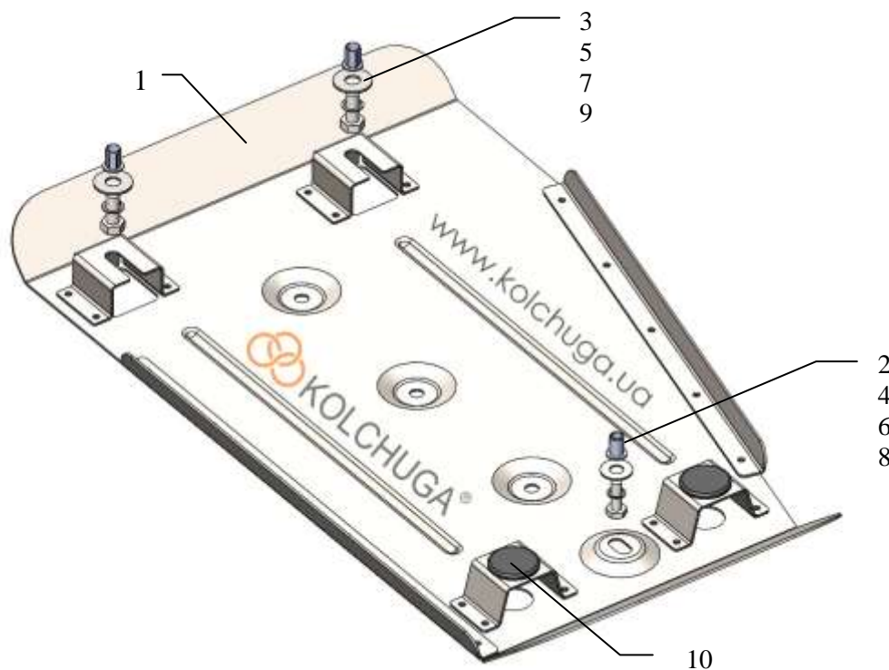
Схема захисту.
